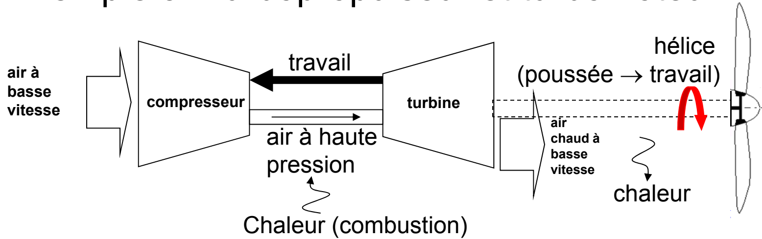
turbopropulseur
