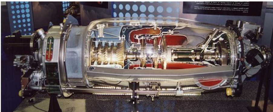
turbopropulseur
